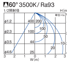
■照明率表 (定格光束 760lm)
