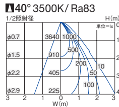
■照明率表 (定格光束 2150lm)
