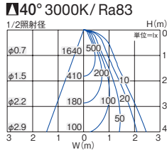
■ 照度率表 (定格光束 960lm)
