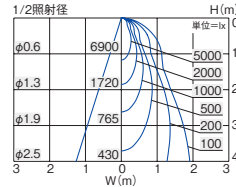
■照明率表 (定格光束 4150lm)
