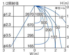
■照明率表 (定格光束 4100lm)
