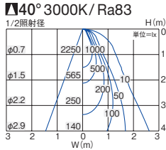
■照明率表 (定格光束 1310lm)
