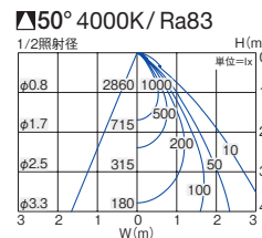
■照明率表 (定格光束 2310lm)
