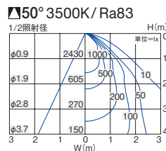
■ 照明率表 (定格光束 3110lm)
