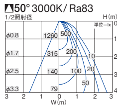
■ 照度率表 (定格光束 1020lm)
