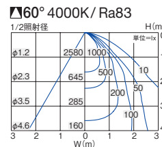
■照明率表 (定格光束 3480lm)
