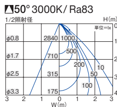
■照明率表 (定格光束 2290lm)
