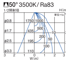
■照明率表 (定格光束 1410lm)
