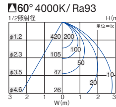
■照明率表 (定格光束 800lm)
