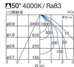
■ 照明率表 (定格光束 3140lm)
