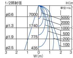
■照明率表 (定格光束 4200lm)
