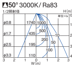
■照明率表 (定格光束 1400lm)
