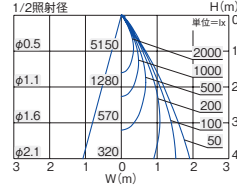
■ 照明率表 (定格光束 1870lm)
