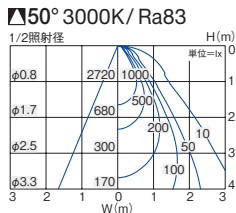
■照明率表 (定格光束 2340lm)
