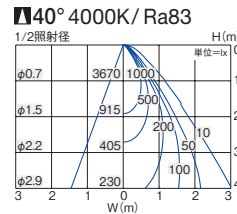
■照明率表 (定格光束 2170lm)
