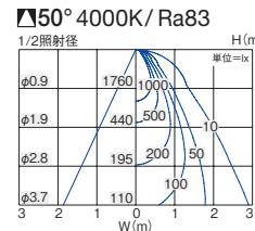
■照明率表 (定格光束 1420lm)
