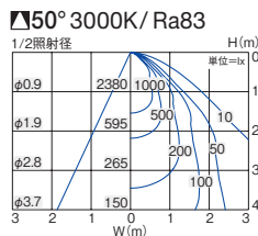
■ 照明率表 (定格光束 3050lm)
