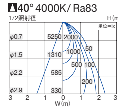
■ 照明率表 (定格光束 3300lm)
