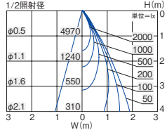
■ 照明率表 (定格光束 1810lm)
