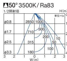
■照明率表 (定格光束 2300lm)
