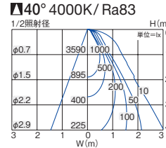
■照明率表 (定格光束 2230lm)
