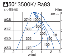
■照明率表 (定格光束 2360lm)
