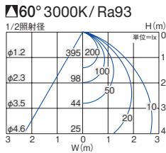
■照明率表 (定格光束 750lm)
