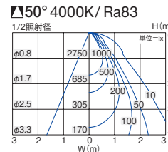
■照明率表 (定格光束 2370lm)
