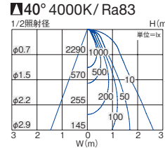
■照明率表 (定格光束 1330lm)
