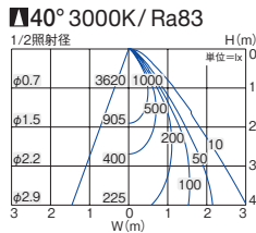
■照明率表 (定格光束 2140lm)
