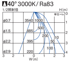
■照明率表 (定格光束 2200lm)
