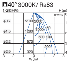
■ 照明率表 (定格光束 3210lm)
