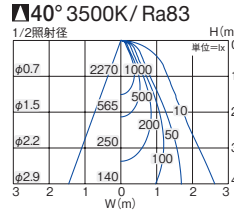
■照明率表 (定格光束 1320lm)
