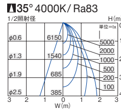
■照明率表 (定格光束 3460lm)
