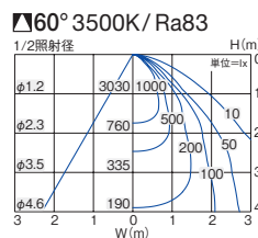
■ 照明率表 (定格光束 4100lm)
