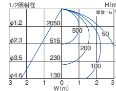
■照明率表 (定格光束 5300lm)
