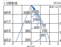
■ 照明率表 (定格光束 2030lm)
