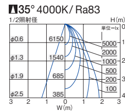
■ 照明率表 (定格光束 3460lm)
