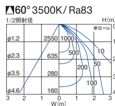
■ 照明率表 (定格光束 3440lm)
