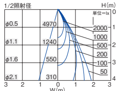
■ 照明率表 (定格光束 1810lm)
