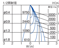
■照明率表 (定格光束 2780lm)
