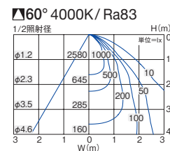
■ 照明率表 (定格光束 3480lm)
