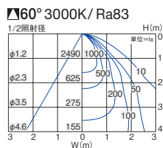
■ 照明率表 (定格光束 3370lm)
