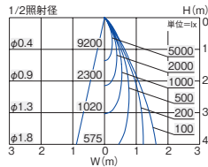
■照明率表 (定格光束 2620lm)
