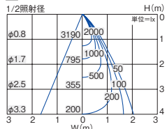
■ 照明率表 (定格光束 1970lm)
