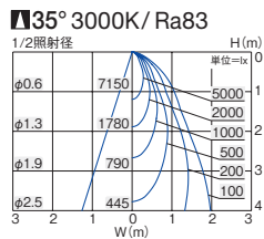
■ 照明率表 (定格光束 4000lm)
