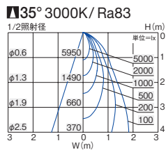
■ 照明率表 (定格光束 3350lm)
