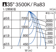
■ 照明率表 (定格光束 4050lm)
