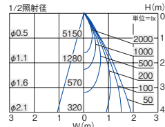
■ 照明率表 (定格光束 1870lm)
