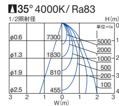
■ 照明率表 (定格光束 4100lm)
