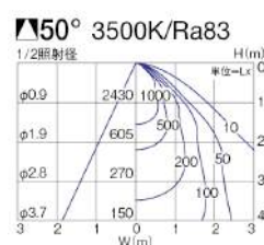
■照明率表 ( 定格光束 3110lm)
