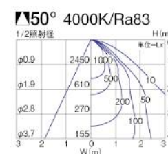
■照明率表 ( 定格光束 3140lm)
