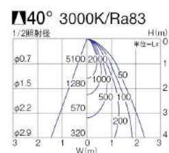
■照明率表 ( 定格光束 3210lm)
