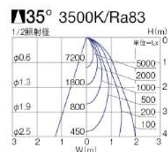
■照明率表 ( 定格光束 4050lm)
