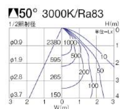
■照明率表 ( 定格光束 3050lm)
