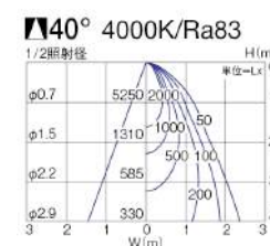
■照明率表 ( 定格光束 3300lm)
