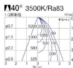
■照明率表 ( 定格光束 3270lm)
